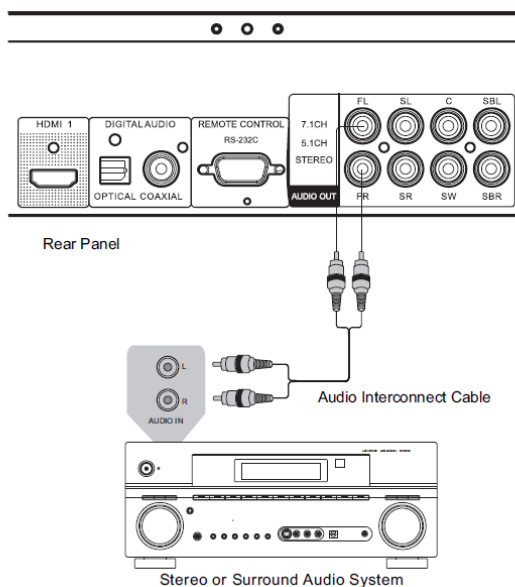
Metodo 8 – Collegamento audio stereo analogico
