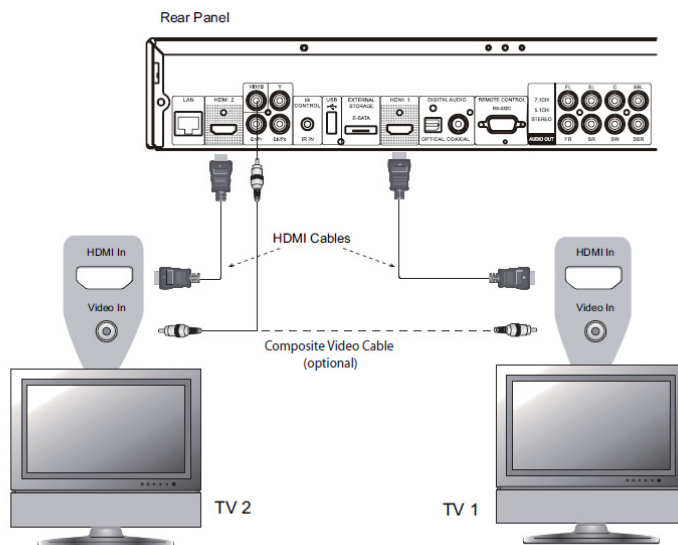
Metodo 2 – Collegamento diretto a due TV via HDMI
