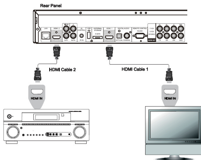
Metodo 9 – Collegamento Dual HDMI
