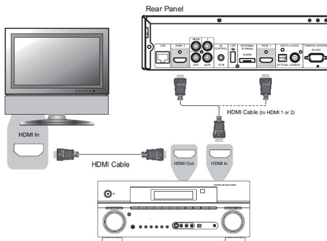
Metodo 5 – collegamento a ricevitore e TV via HDMI
