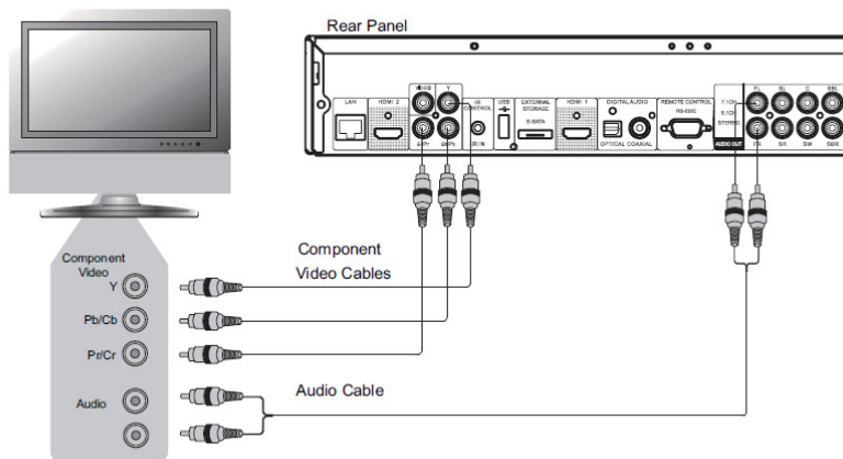
Metodo 4 – collegamento video Component al TV
