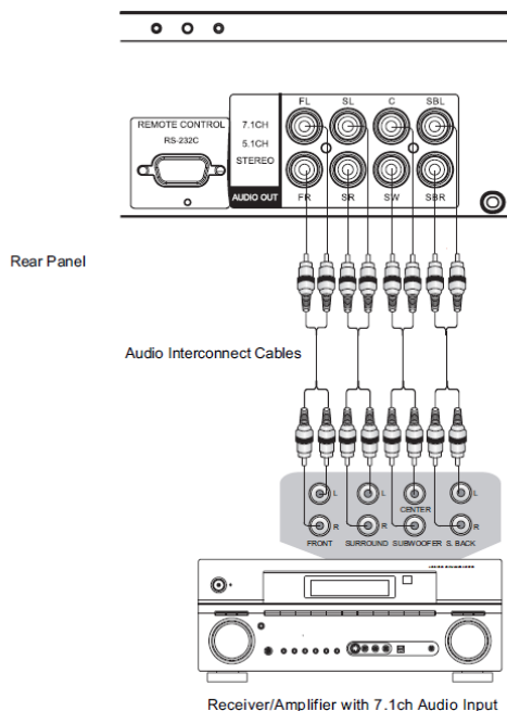
Metodo 6 – collegamento audio analogico 7.1ch
