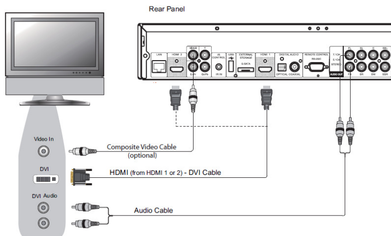
Metodo 3 – collegamento DVI al TV
