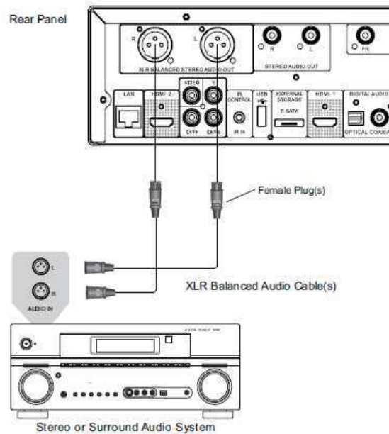
Methode 9 – Analoger Stereo-Anschluss über XLR-Kabel
