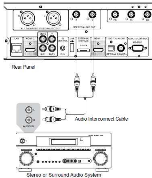
Methode 8 –Analoger Stereo-Anschluss über Cinch-Kabel
