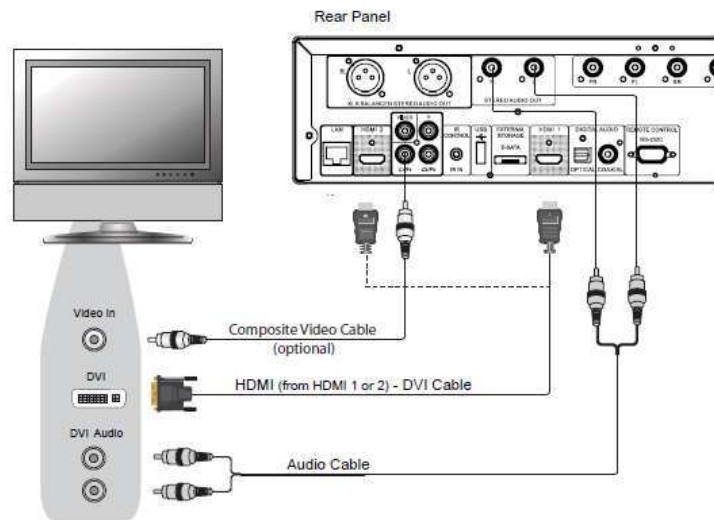
Methode 3 – DVI-Eingang am TV-Gerät
