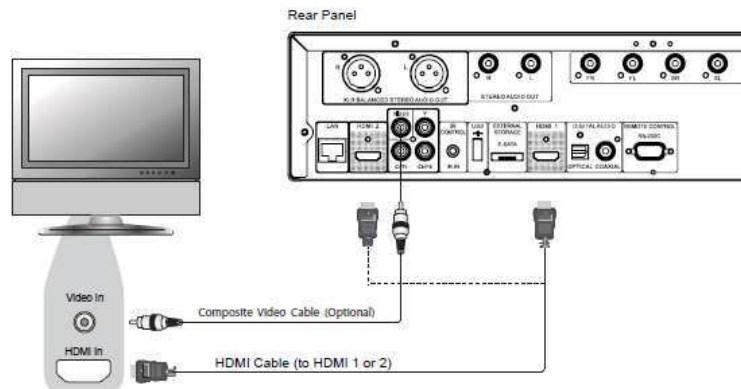
Methode 1 – Direkte HDMI-Verbindung an ein einzelnes TV-Gerät
