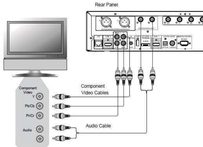
Methode 4 – Komponentenvideoverbindung zu einem TV
