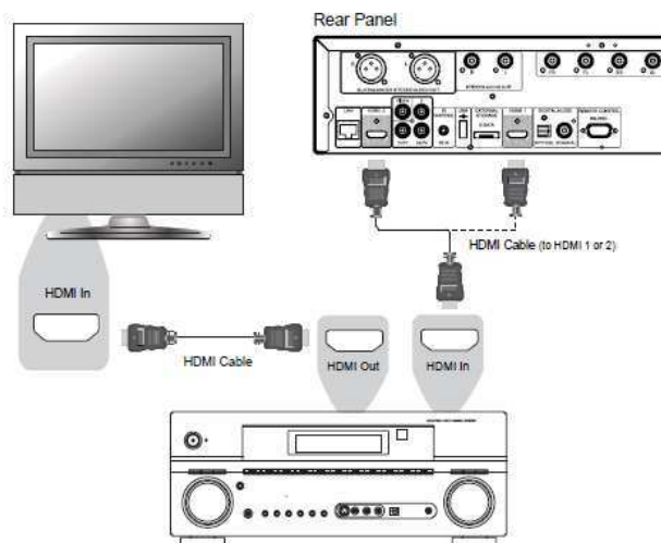
Methode 5 – HDMI-Verbindung zu einem Receiver und an ein TV-Gerät
